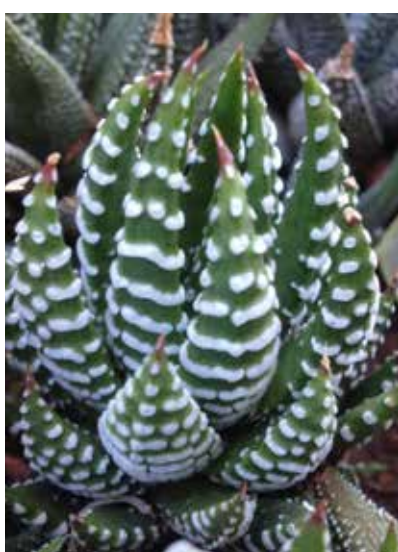
HAWORTHIA COARCTATA 86283
